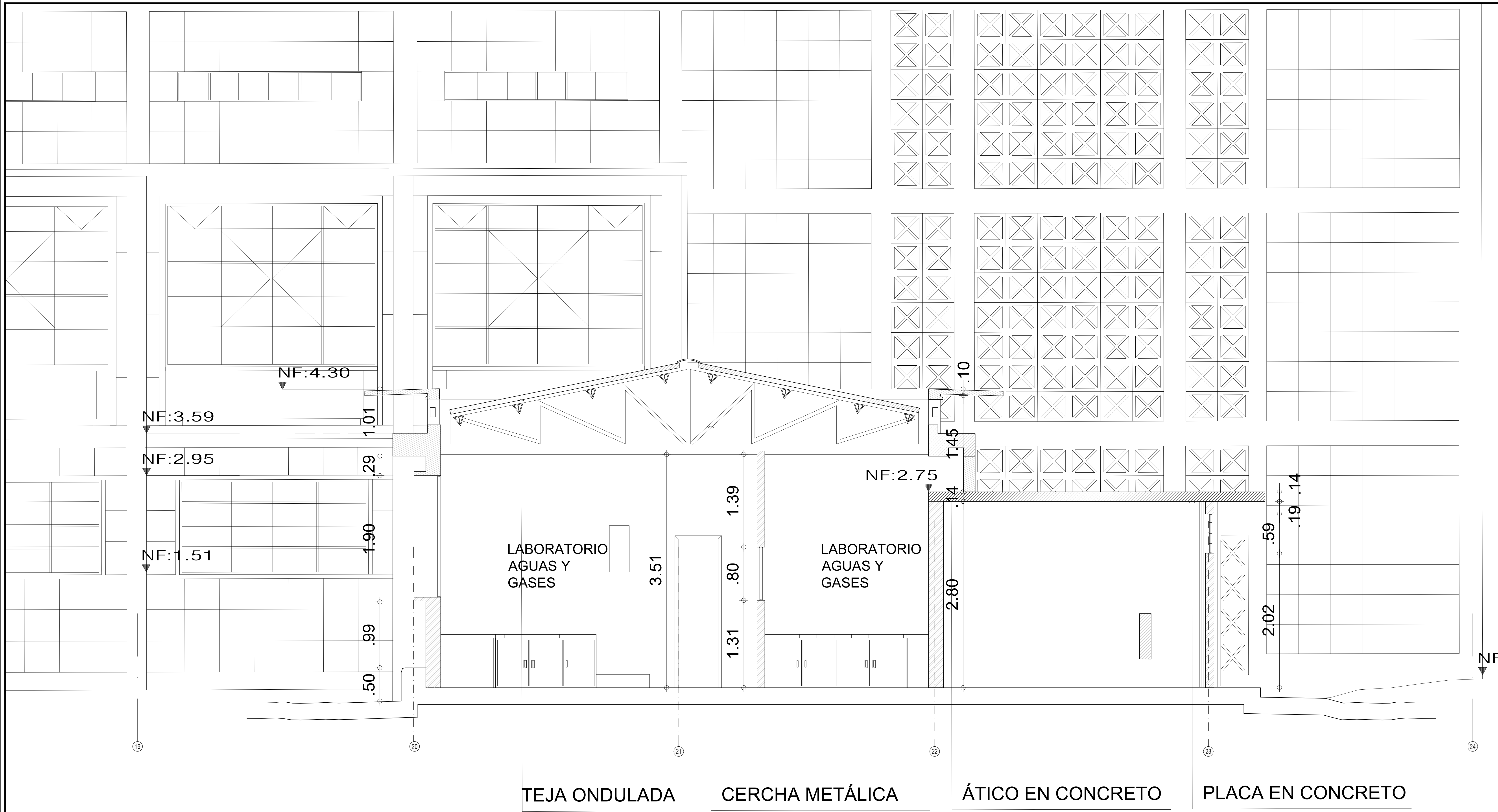
CORTE DL-01 ESCALA 1:25
